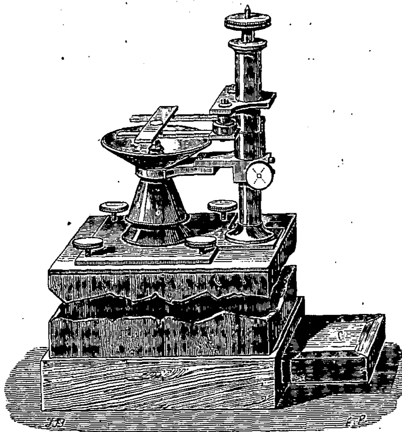
Fig. 14. — Microscope photographique.
