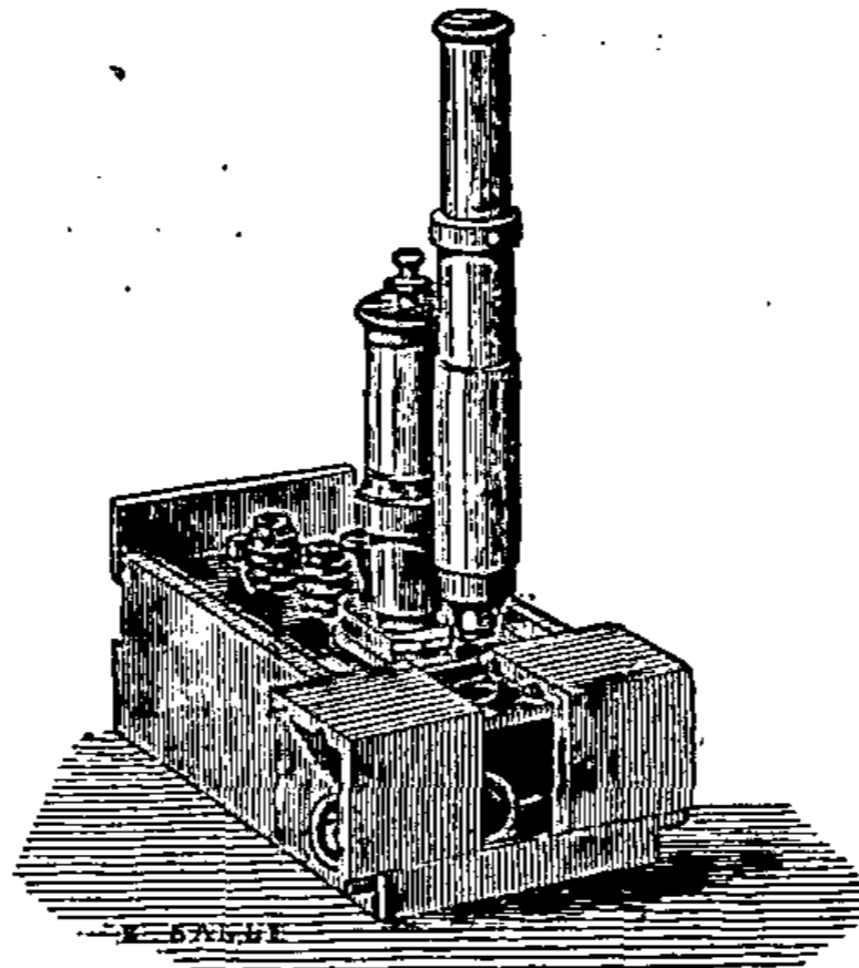
Fig. 8. — Microscope portatif monté, de Nacet.
